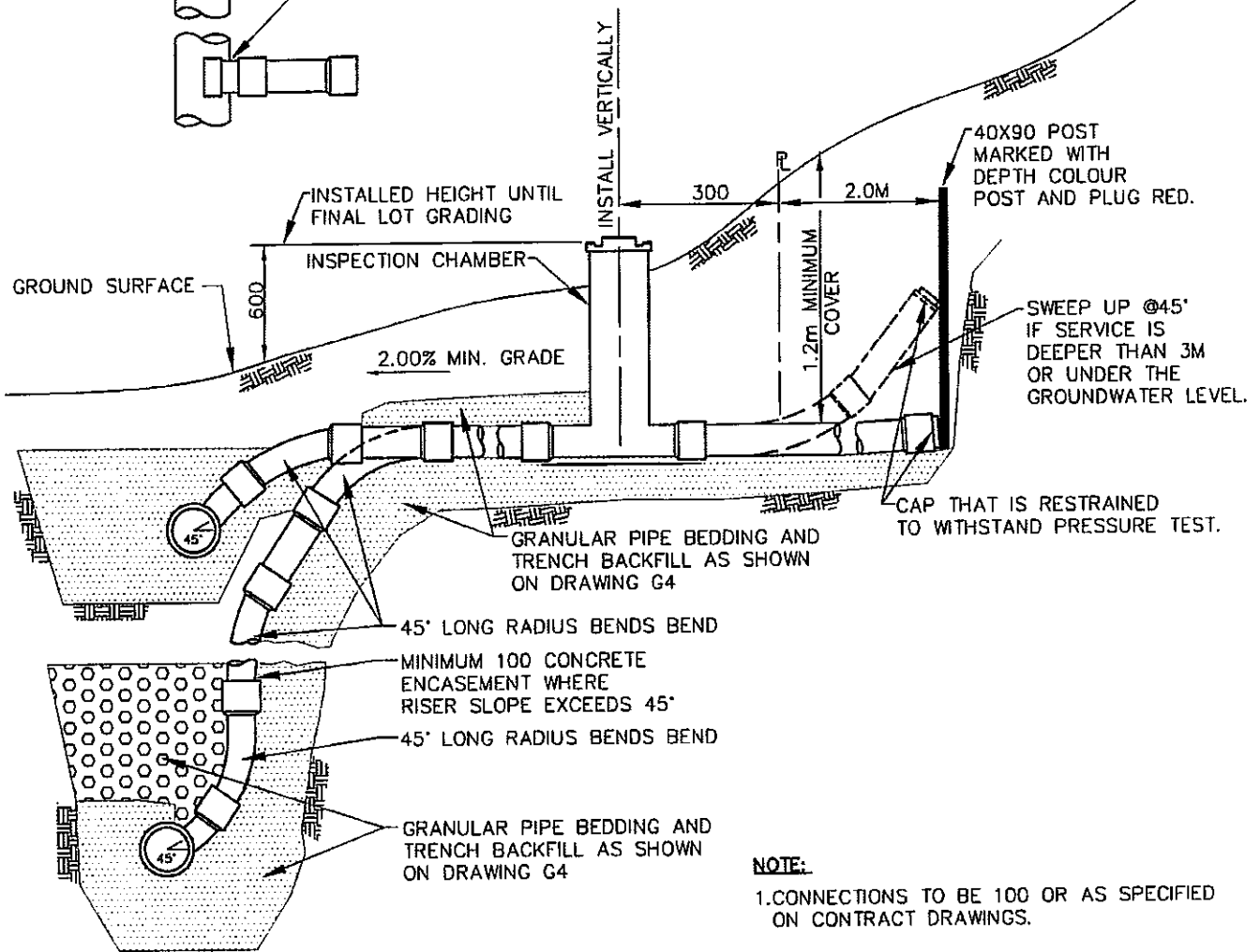
ELEVATION N.T.S
